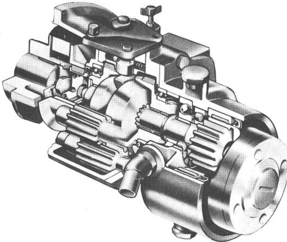
Reverse Gear type Mono Shift (MSB).
